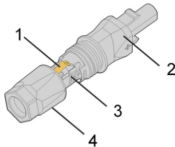
Abbildung 4-1 Komponenten des SUNCLIX-Steckverbinders
